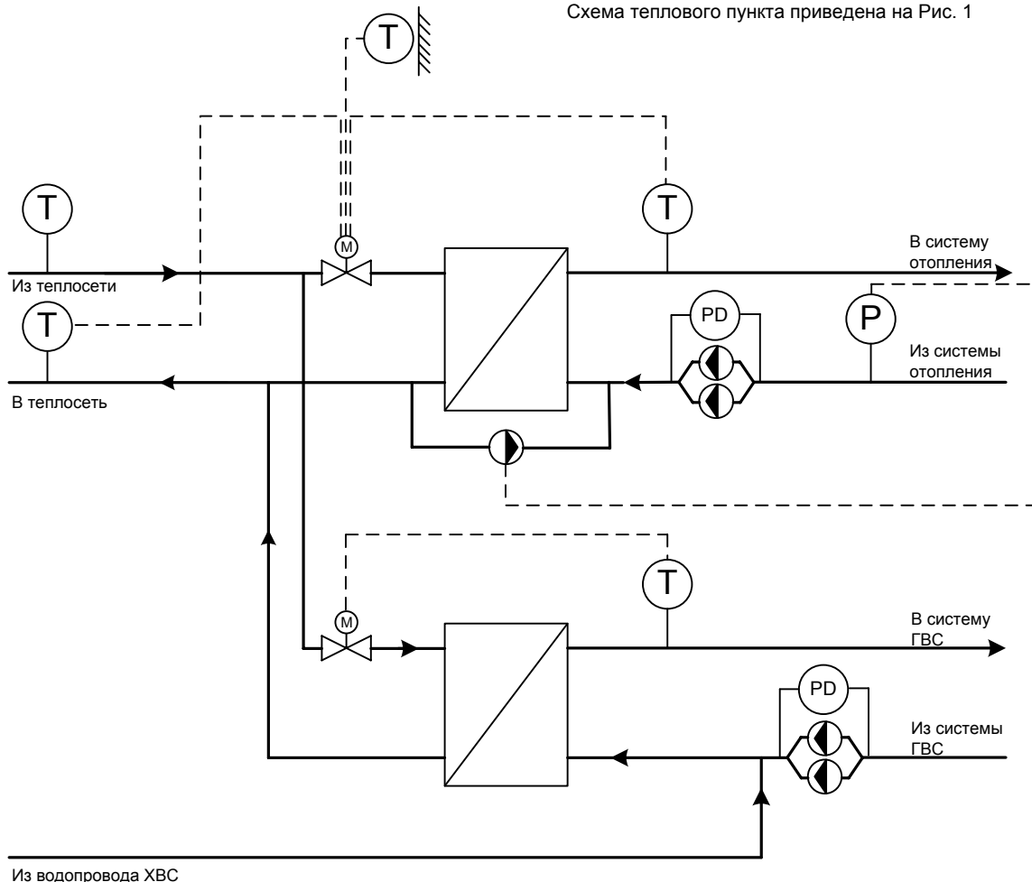
Рис. 1 – Схема ИТП
