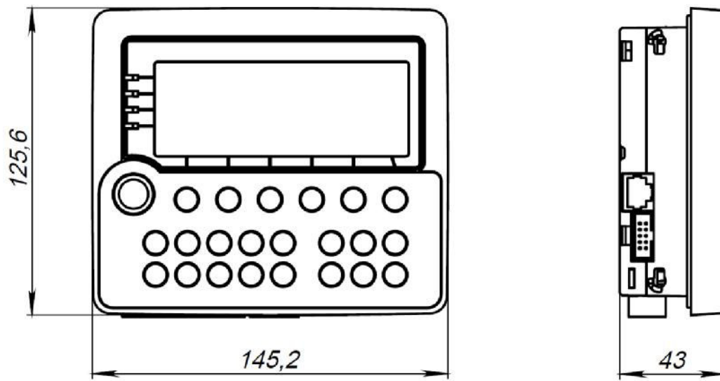
Габаритные размеры прибора с подключенным «МС»
