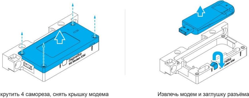
Рис. 5 – Извлечение заглушки разъема антенны
