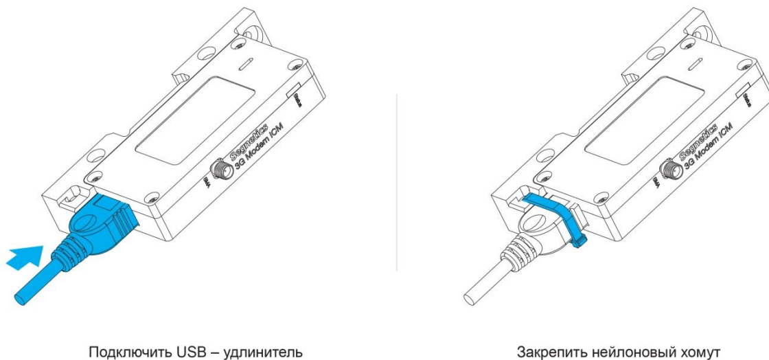
Рис. 10 – Фиксация USB-удлинителя
