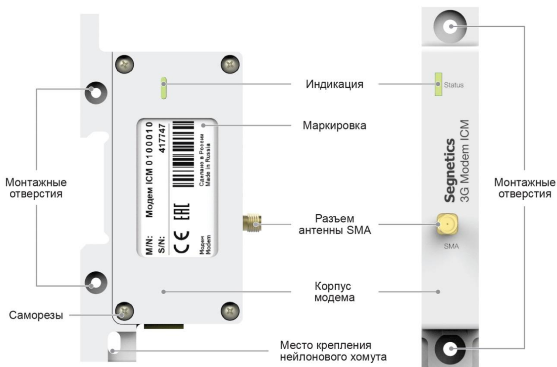
Рис. 1 – Основные части модема
