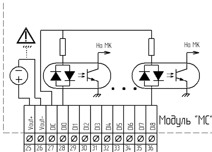
Рисунок 12. Упрощенная электрическая принципиальная схема цифровых входов МС. D1C – общая клемма, D1x – вход двунаправленного оптрона, Vout+ Vout- - выходы внутреннего источника напряжения цифровых входов.
