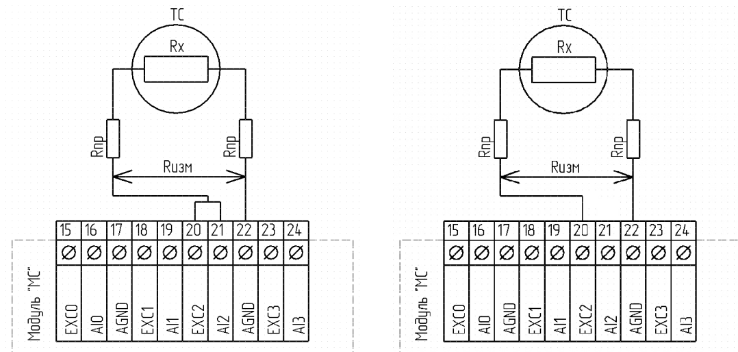
Рисунок 23. Схемы двухпроводного подключения резистивных датчиков
