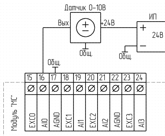
Рисунок 21. Пример подключения датчика с выходом «0-10В»
